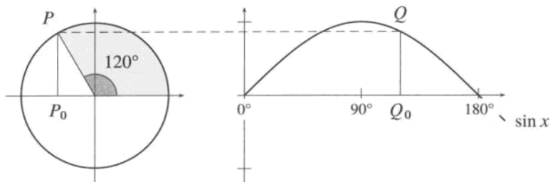
图 5.18 正弦函数与单位圆 (PSTricks 实现)
