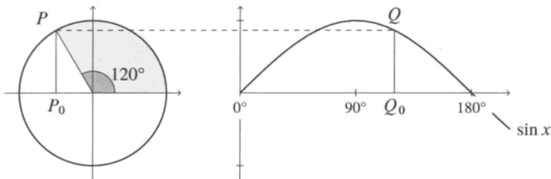
图 5.19 正弦函数与单位圆 (TikZ 实现)
